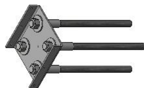
BULTGRUPP ( 1 : 5 )
