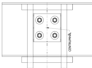
UTSÄTTNING ( 1 : 5 )
