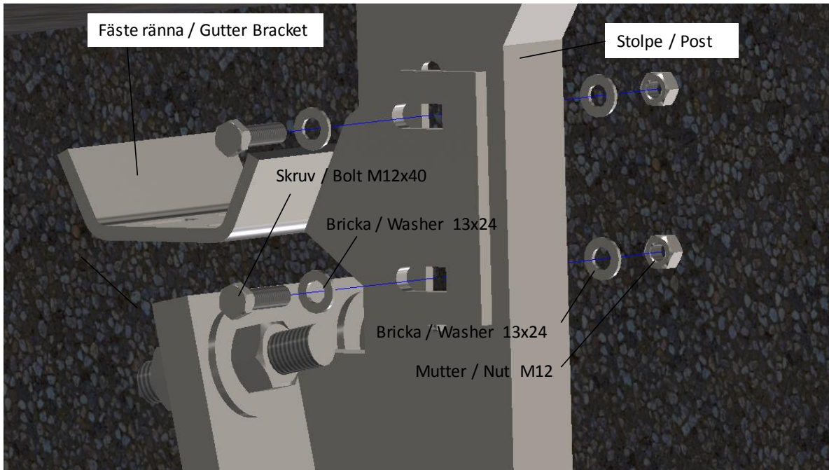
Fäste ränna
